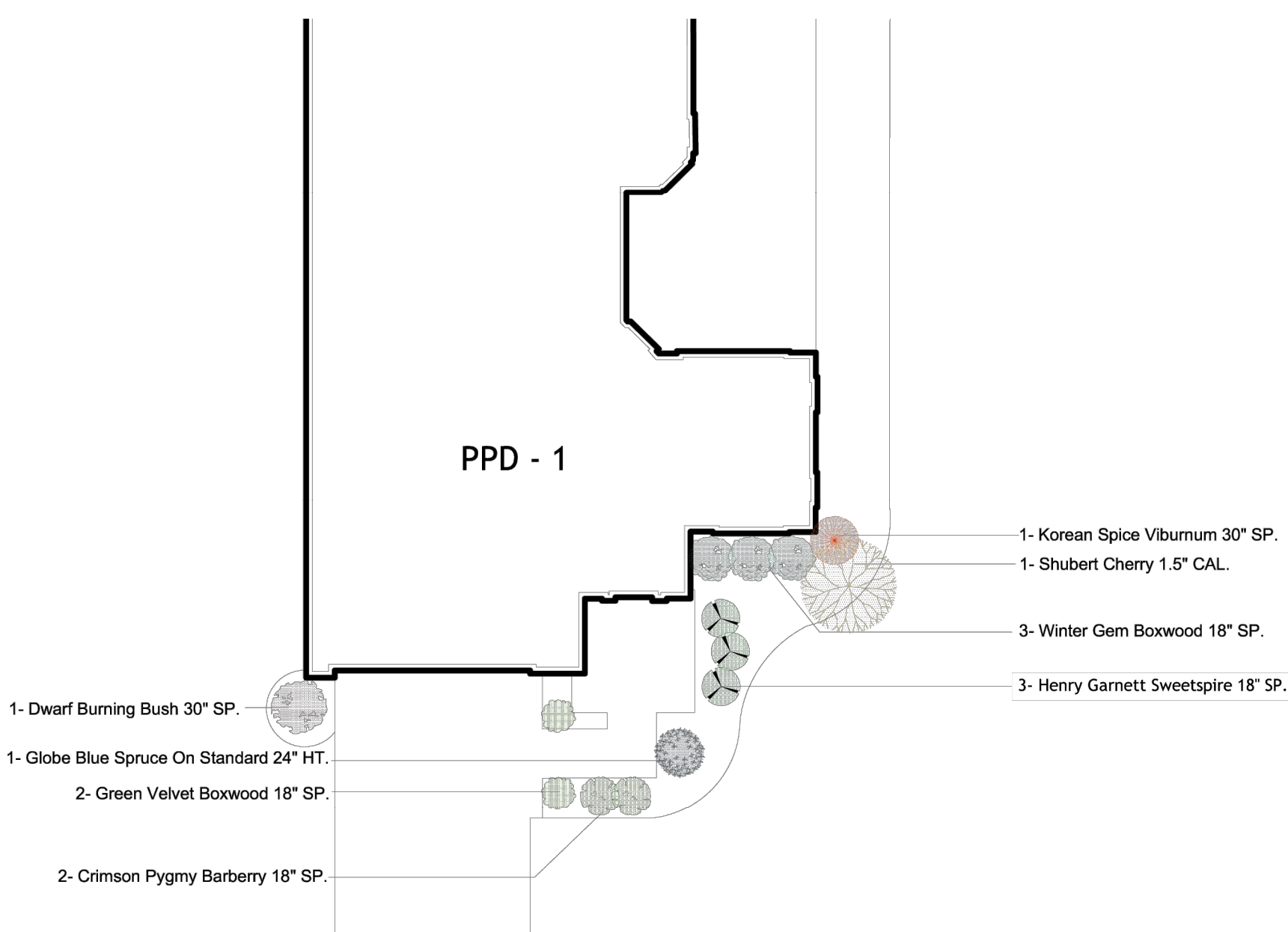
⑤ PALAZZO (D-1) TYPICAL FRONT LANDSCAPE PLAN SCALE: N.T.S.
